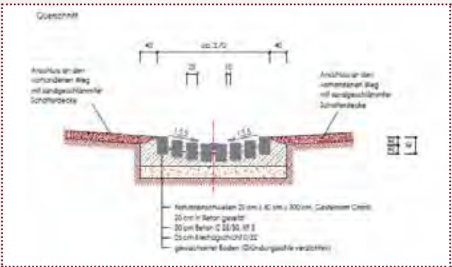
Querschnitt Furt, Offenlegung Weißiger Bach, Quelle: ÖkoProjekt ElbeRaum GmbH Dresden
