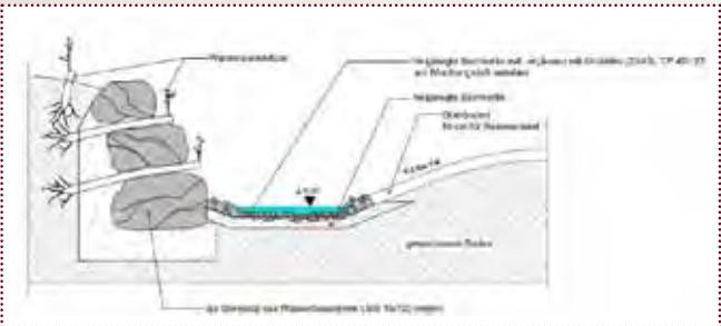
Konstruktionsdetail Böschungsbefestigung Quelle: Ausführungsplanung, Planungsbüro Schubert, Radeberg
