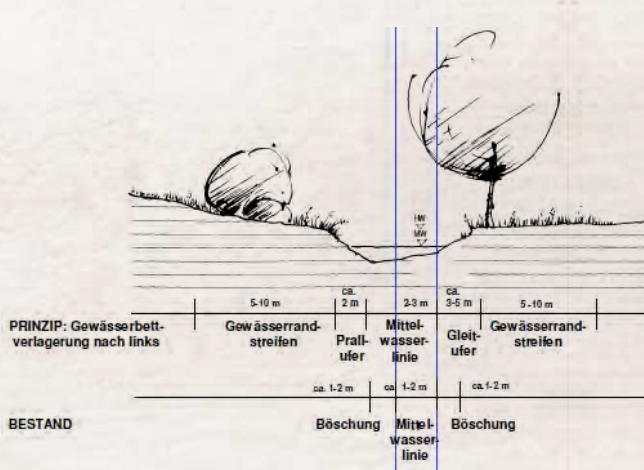
Aufwertung und leichte Gewässerbettverlagerung, Prallufer links Quelle: KÜHFUSS, LandschaftsArchitektur* Umweltplanung Dresden
